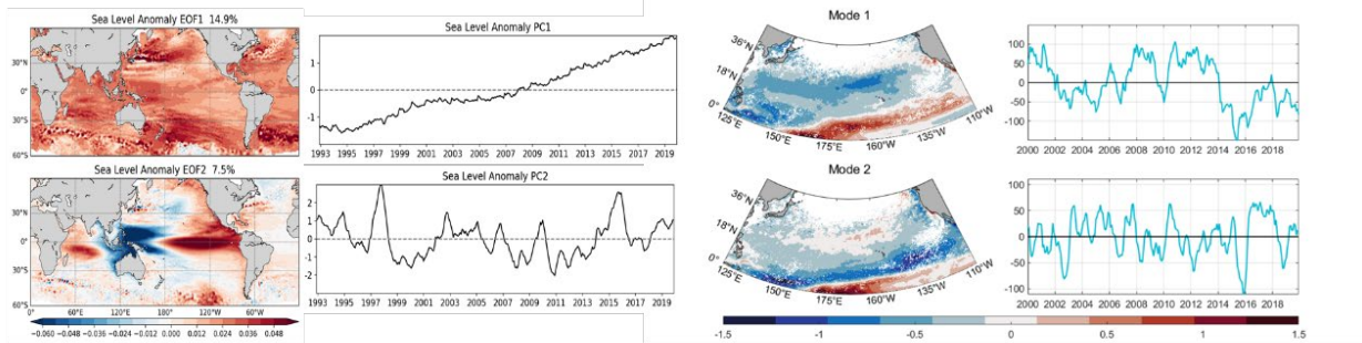
海表面高度EOF分解后的前两个主模态
