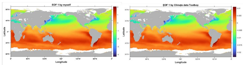
海表面温度经不同EOF程序分解的第一模态对比
